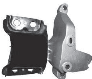
Código: 80203 HIDRAULICO Modelo: KANGOO K9K-CLIO II-SYMBOL II Nº Original: 8200410267 Soporte de motor derecho
