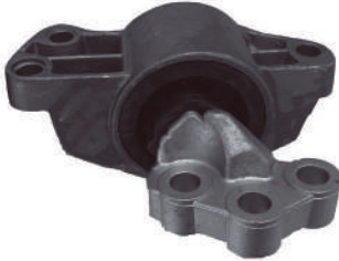
Código: 50194 Modelo: UNO NOVO-PUNTO Nº Original: 51879121 Soporte de motor derecho
