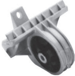
Código: 80120 Modelo: R. 19 - CLIO Nº Original: 7700804163 Soporte central de motor
