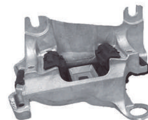
Código: 80197 Modelo: FLUENCE-MEGANE III CAJA AUTOMATICA Nº Original: 112206677R Soporte de motor izquierdo
