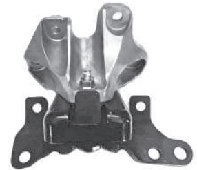
Código: 40075 Modelo: S10 MOTOR 2.4 L Nº Original: 52037204 Soporte de Motor Derecho
