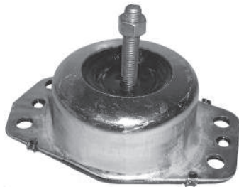
Código: 80156 Modelo: MASTER Nº Original: 8200022595 Soporte de motor derecho
