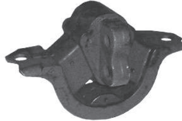
Código: 40027 Modelo: CORSA 1.7 Diesel Nº Original: 93269291 Soporte de motor lado caja
