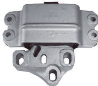
Código: 90081 Modelo: TIGUAN 2009 EN ADELANTE Nº Original: 5N0.199.155 Soporte de motor izquierdo
