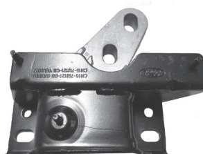
Código: 70224 Modelo: ECOSPORT KINETIC 2.0 4X2 Nº Original: CN15-7M121-CB Soporte de motor izquierdo
