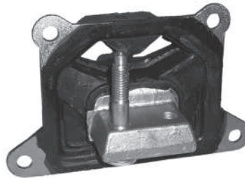
Código: 40033 Modelo: CORSA Nº Original: 90445300 Soporte de motor derecho nafta con aire
