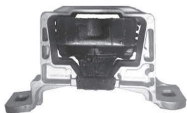
Código: 70216 HIDRAULICO Modelo: FOCUS II SIGMA 1.6 09.. Nº Original: 3M51-6F012-CJ Soporte de motor derecho hidraulico
