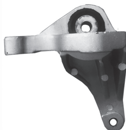
Código: 70237 Modelo: FOCUS 2 1.8 DIESEL Nº Original: 3M516P093AE Soporte de caja de velocidades
