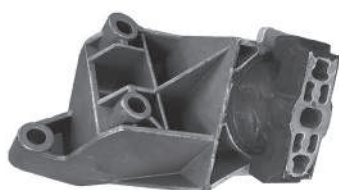
Código: 80200 Modelo: TWINGO Nº Original: 7700412094 Soporte de motor derecho
