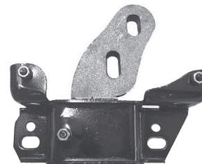
Código: 70230 Modelo: ECOSPORT KINETIC 4X2 13 Nº Original: CV21-7M121-AC Soporte de motor izquierdo
