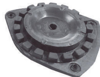
Código: 80195 Modelo: FLUENCE-MEGANE III Nº Original: 54320001R Soporte de amortiguador
