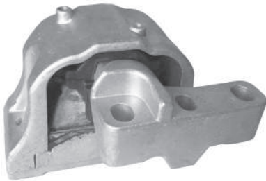
Código: 90046 HIDRAULICO Modelo: GOLF 1.8 - BORA - PASSAT - A3 Nº Original: 1J0.199.262.BF Soporte motor hidráulico lado derecho
