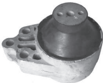
Código: 70166 HIDRAULICO Modelo: FOCUS - FIESTA - ECOSPORT Nº Original: 2N15-6F012-JB Soporte motor hidráulico lado derecho
