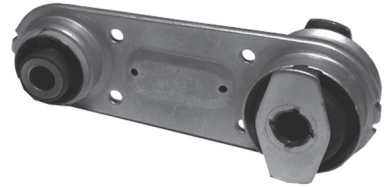
Código: 80217 Modelo: LAGUNA 2 Nº Original: 8200371093 Soporte de motor trasero
