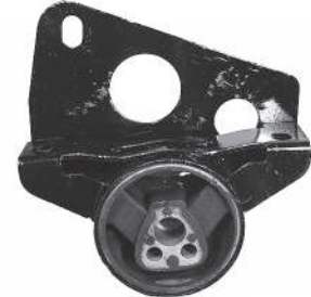
Código: CH202 Modelo: QQ 2008/2015 Nº Original: S11-1001310-BA Soporte de motor derecho
