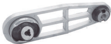
Código: 80205 Modelo: LOGAN-MEGANE-SANDERO-SCENIC-CLIO III Nº Original: 8200500928 Soporte de motor trasero central reforzado
