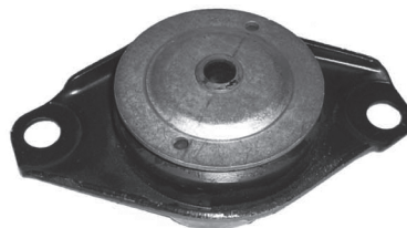
Código: 50159 Modelo: PALIO 1.8 Nº Original: 0051715728 Soporte de caja de velocidades
