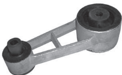
Código: 80136 Modelo: KANGOO 1.9 Diesel Nº Original: 7700426193 Soporte de motor lado caja
