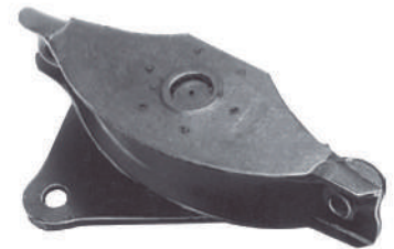
Código: 50016 Modelo: FIAT 128 Nº Original: 4218081 Soporte de motor 1300 (lado caja)
